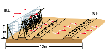
図2 防風ネットの設置
