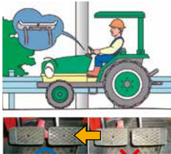
図2：道路走行時の左右ブレーキ連結 出典：農研機構ホームページより
